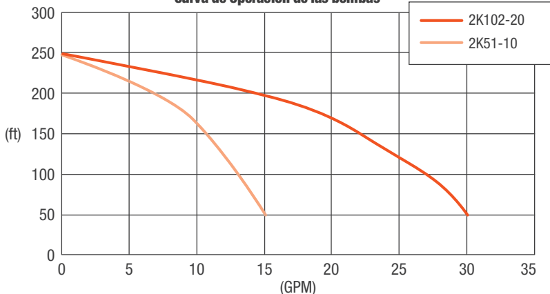
Curva de Operación de las bombas
