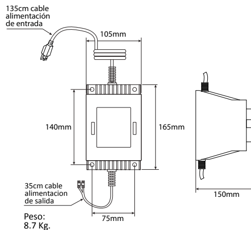
CÓDIGO: TRAFO-500-12A
