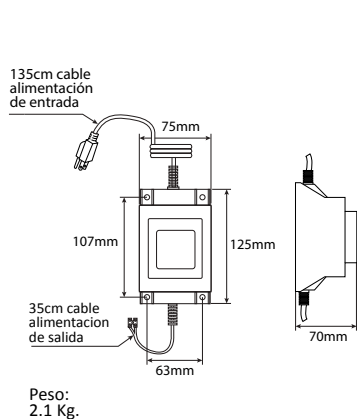
CÓDIGO: TRAFO-100-12A
